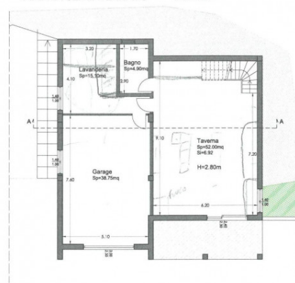
PIANTA SEMINTERRATO scala 1:100
